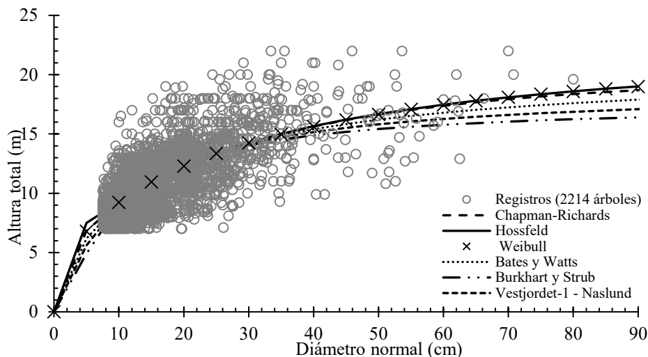
FIGURA. 2. Modelos locales altura total-diámetro normal ( A-d ) ajustados para Lysiloma latissiliquum en Quintana Roo, México.
