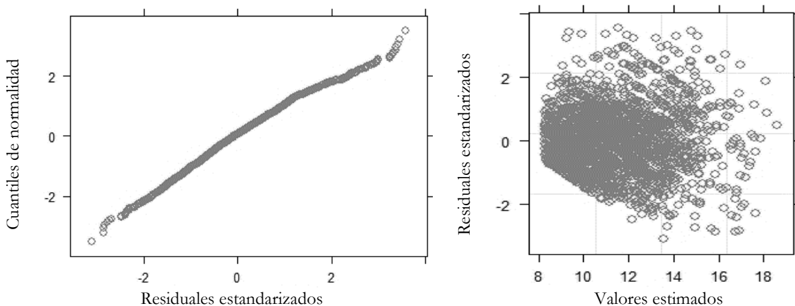
FIGURA. 3. Pruebas gráficas de normalidad (a) y homoscedasticidad (b) del modelo Hossfeld (1822) altura total-diámetro normal (A-d) para Lysiloma latisiliquum en Quintana Roo, México.
