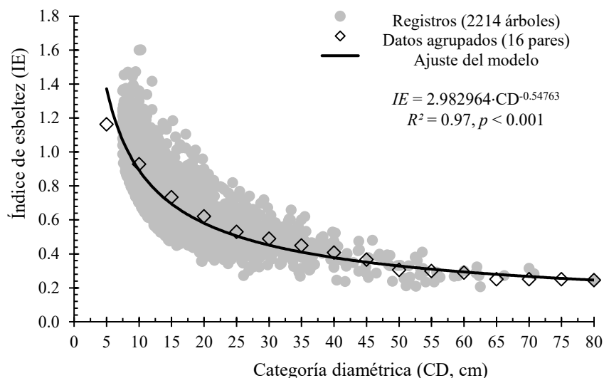
FIGURA. 1. Relación entre índice de esbeltez ( IE : Altura total/diámetro normal) y categoría diamétrica ( CD ) para árboles de Lysiloma latisiliquum en Quintana Roo, México.
