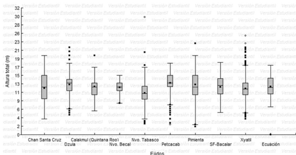
FIGURA. 4. Comparación de medias a 99% de confiabilidad (prueba de t ) entre datos independientes (nueve ejidos) y el modelo 3.2 Hossfeld altura total-diámetro normal (A-d) ajustados para Lysiloma latisiliquum en Quintana Roo, México.
