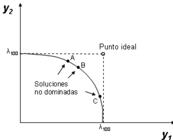
Figura 2. Representación del punto ideal y de las soluciones no dominadas para dos objetivos ( y_1 , y_2 ). Los puntos A, B y C son las soluciones no dominadas y juntas forman la línea conocida como frontera eficiente . El punto B es el más cercano al punto ideal y por lo tanto el que más satisface el conjunto de soluciones óptimas.
